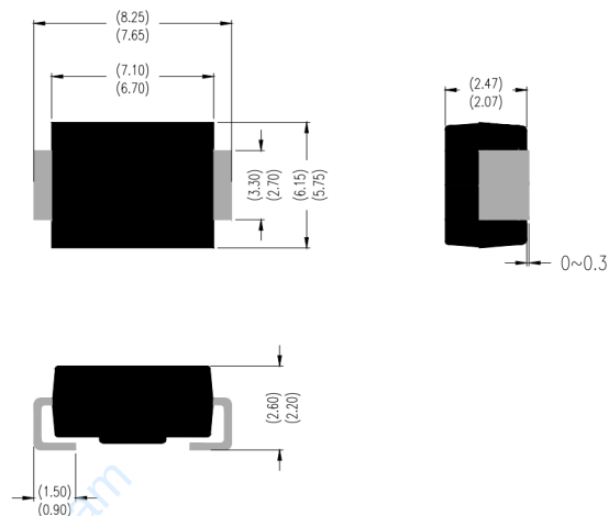
DO-214AB (SMC)
