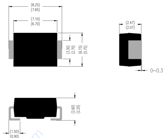
DO-214AB (SMC)
